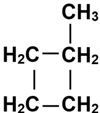
1-метилциклобутан
